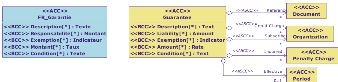
Diagramme de classe : Vue Garantie
