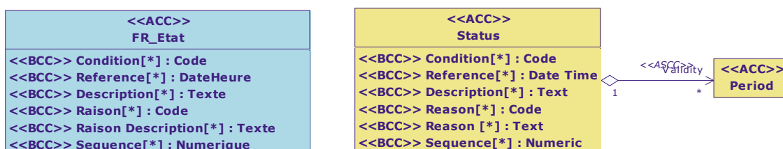
Diagramme de classe : Vue Etat
