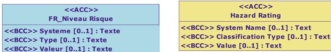
Diagramme de classe : Vue Niveau Risque
