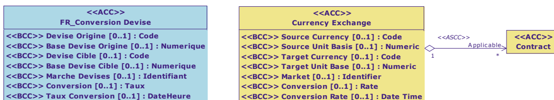
Diagramme de classe : Vue Conversion Devise
