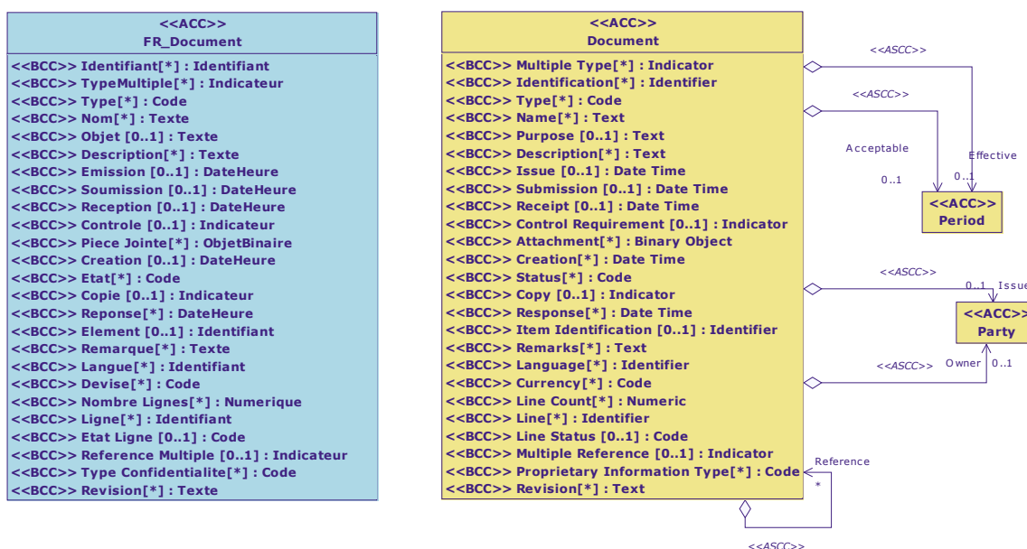
Diagramme de classe : Vue Document
