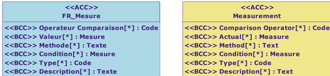
Diagramme de classe : Vue Mesure
