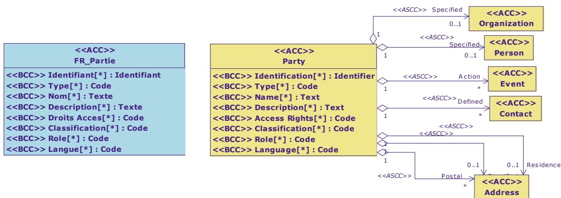
Diagramme de classe : Vue Partie
