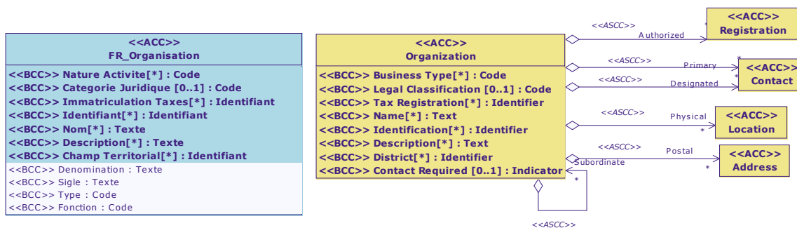
Diagramme de classe : Vue Organisation
