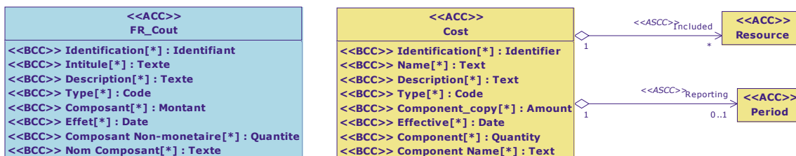
Diagramme de classe : Vue Coût
