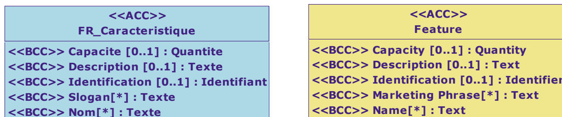
Diagramme de classe : Vue Caracteristique
