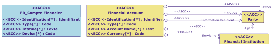
Diagramme de classe : Vue Compte Financier
