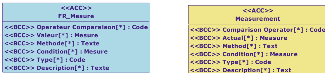
Diagramme de classe : FR_Measurement
