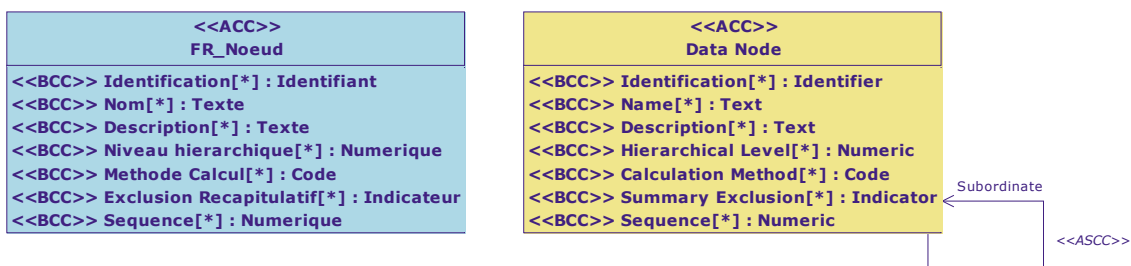
Diagramme de classe : Vue Noeud
