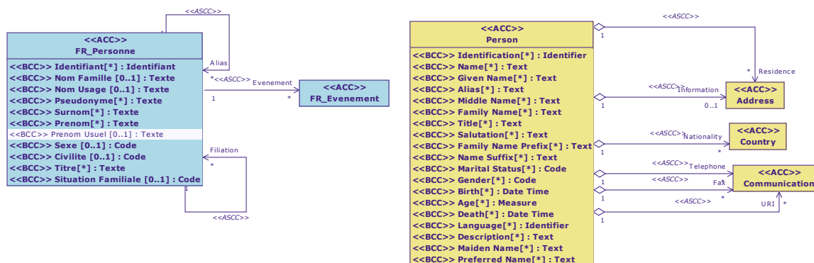
Diagramme de classe : Vue Personne
