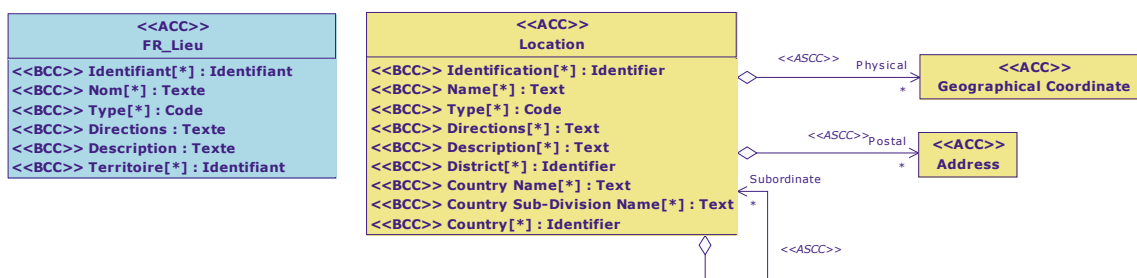
Diagramme de classe : Vue Lieu
