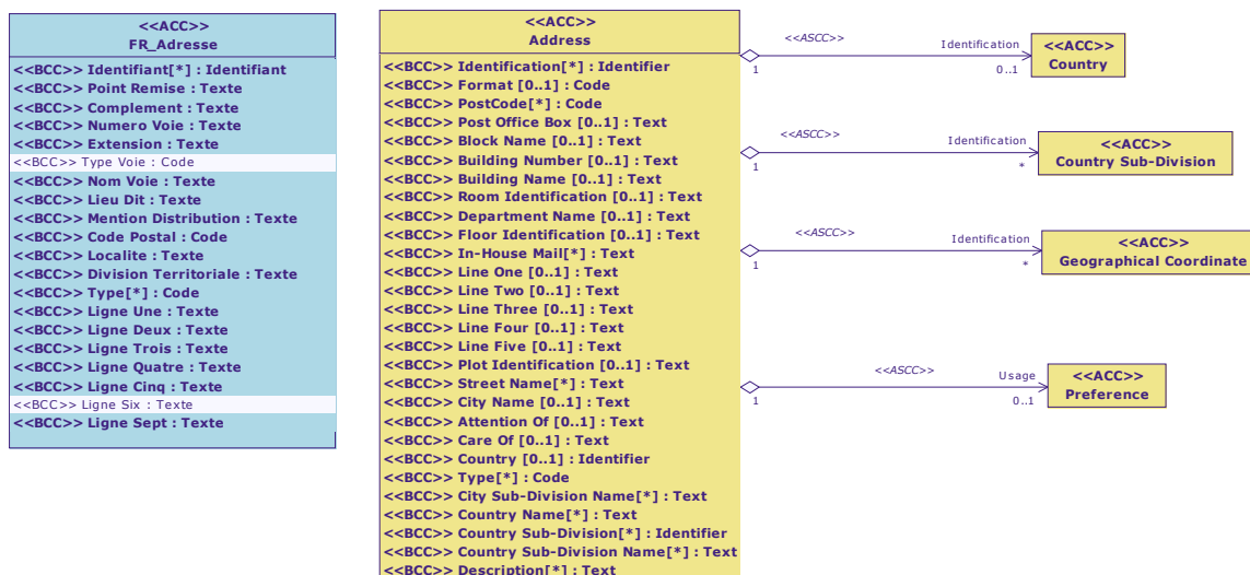
Diagramme de classe : Vue Adresse
