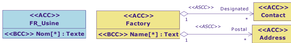
Diagramme de classe : Vue Usine
