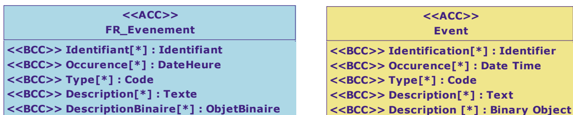
Diagramme de classe : Vue Evènement
