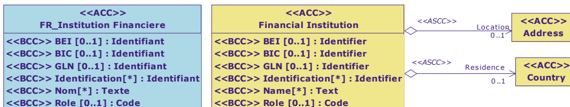
Diagramme de classe : Vue Institution Financiere
