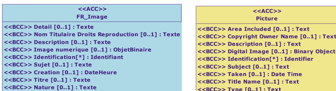
Diagramme de classe : FR_Image
