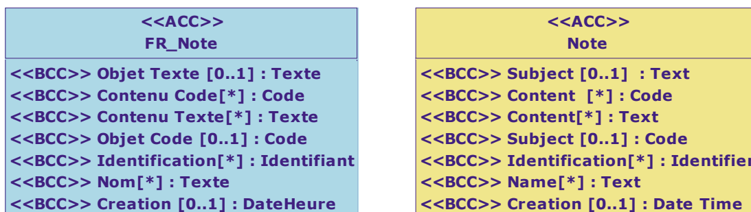
Diagramme de classe : FR_Note
