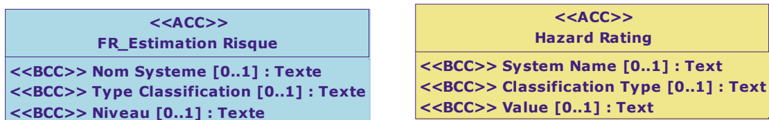
Diagramme de classe : Estimation Risque
