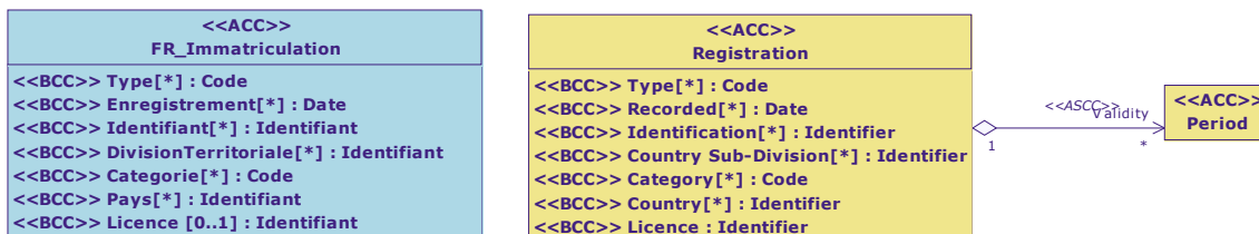
Diagramme de classe : Vue Immatriculation
