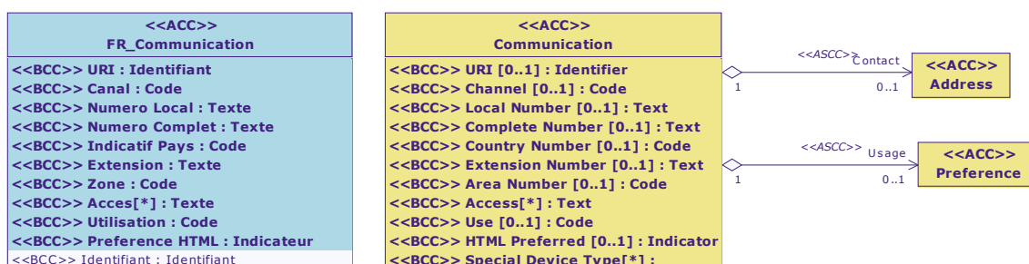
Diagramme de classe : Vue Communication
