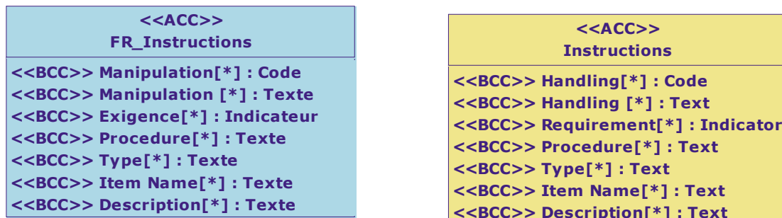
Diagramme de classe : Vue Instructions
