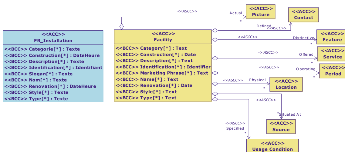
Diagramme de classe : Vue Installation
