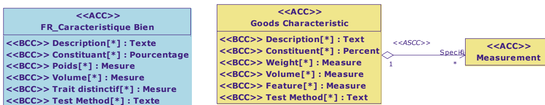
Diagramme de classe : FR_Caractéristique Bien
