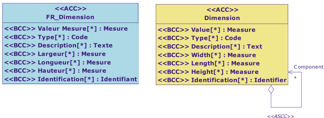
Diagramme de classe : Vue Dimension
