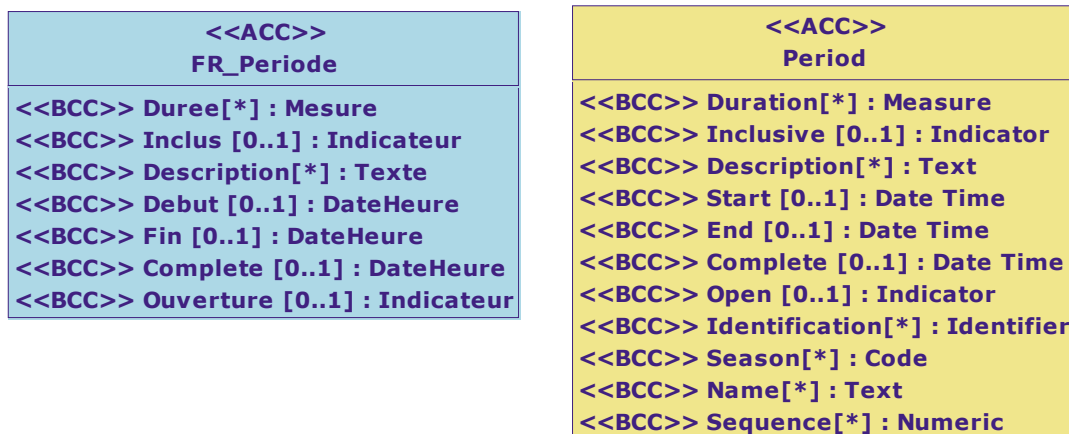
Diagramme de classe : Vue Période
