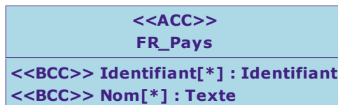
Diagramme de classe : Vue Pays
